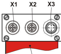
Drehgeber oder Lineargeber / Shaft-Encoder or Linear-Encoder
