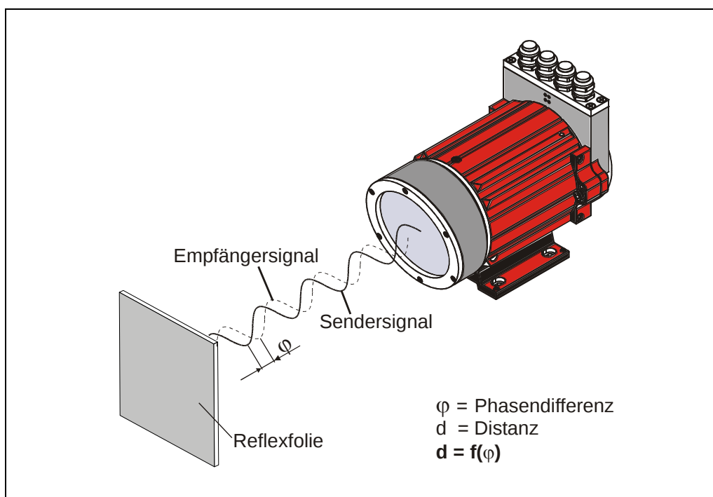
Abbildung 1: Funktionsprinzip
