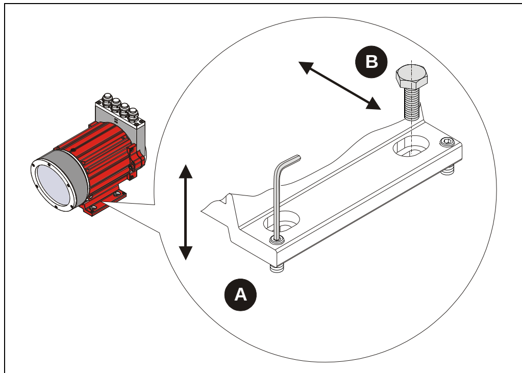
Abbildung 5: Mechanische Justage-Möglichkeiten
