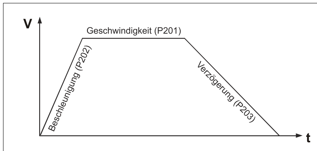
Abbildung 7: Rampeneinstellungen
