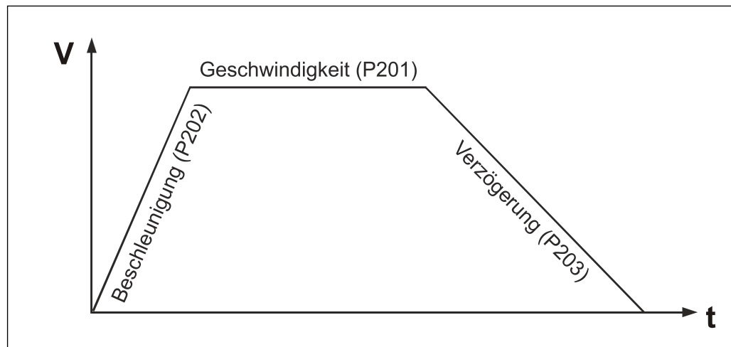
Abbildung 5: Rampeneinstellungen
