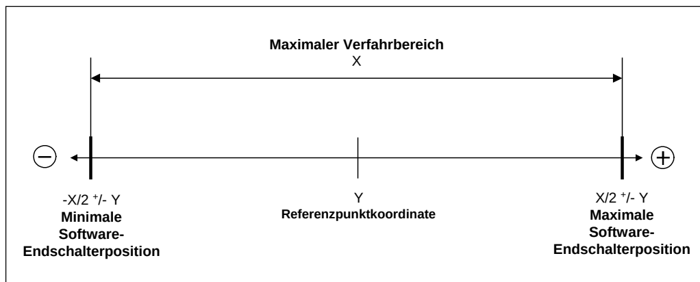
Abbildung 8: Software-Endschalterpositionen / Referenzpunktkoordinate
