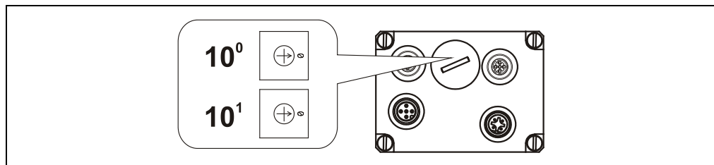
Abbildung 3: EPL Node-ID, Schalterzuordnung
