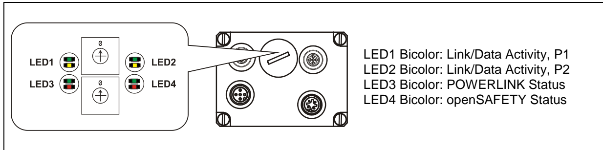
Abbildung 7: Bus-Statusanzeige
