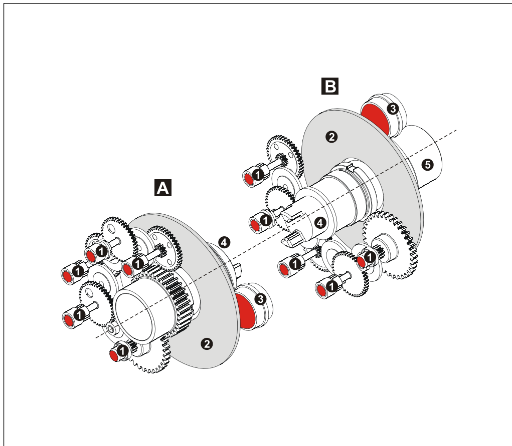
Abbildung 2: Mess-System-Funktionsweise (Doppelabtastung)
