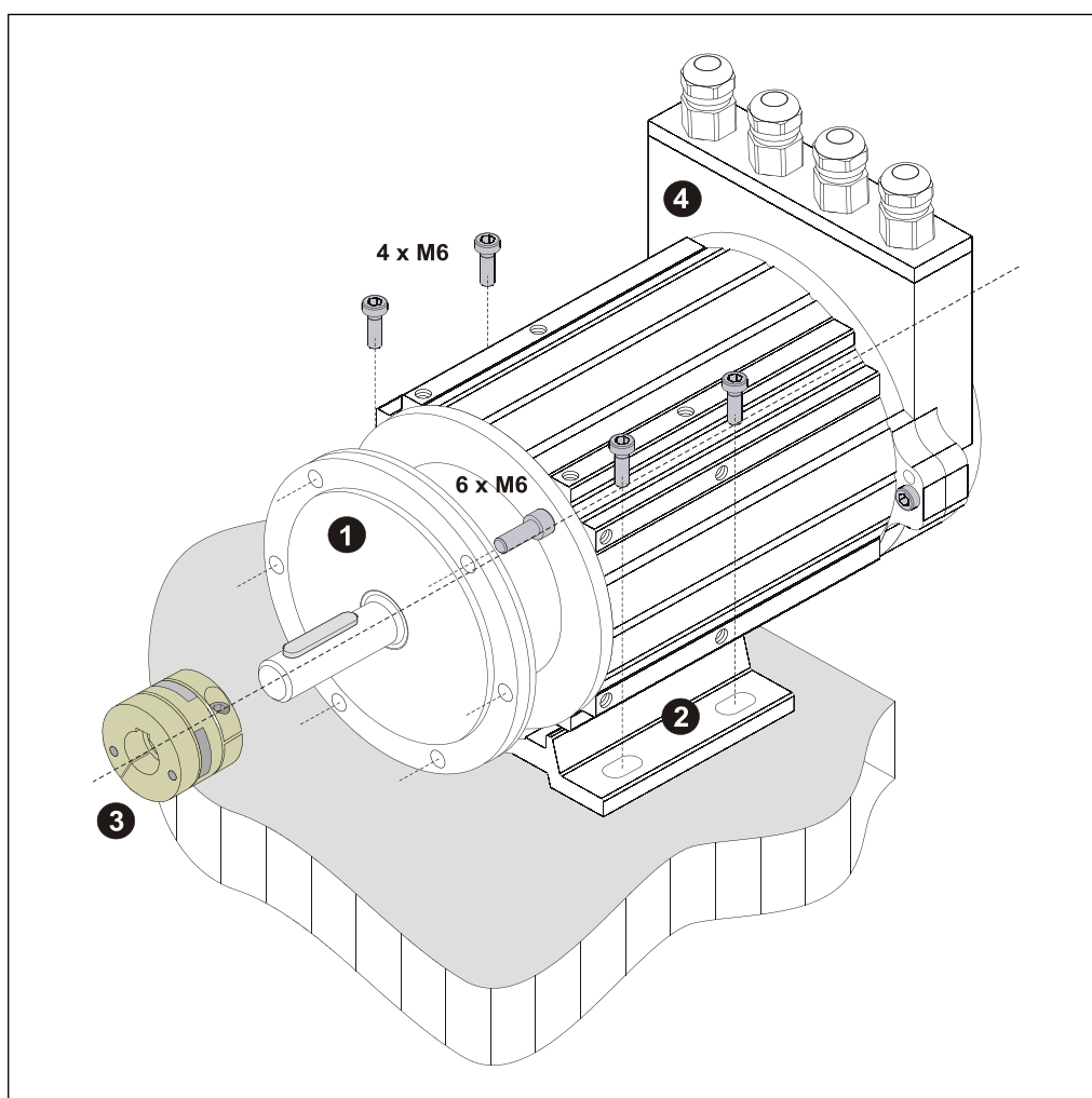
Abbildung 3: Montagebeispiel
