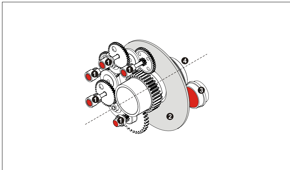
Abbildung 1: Mess-System-Funktionsweise (Einzelabtastung)
