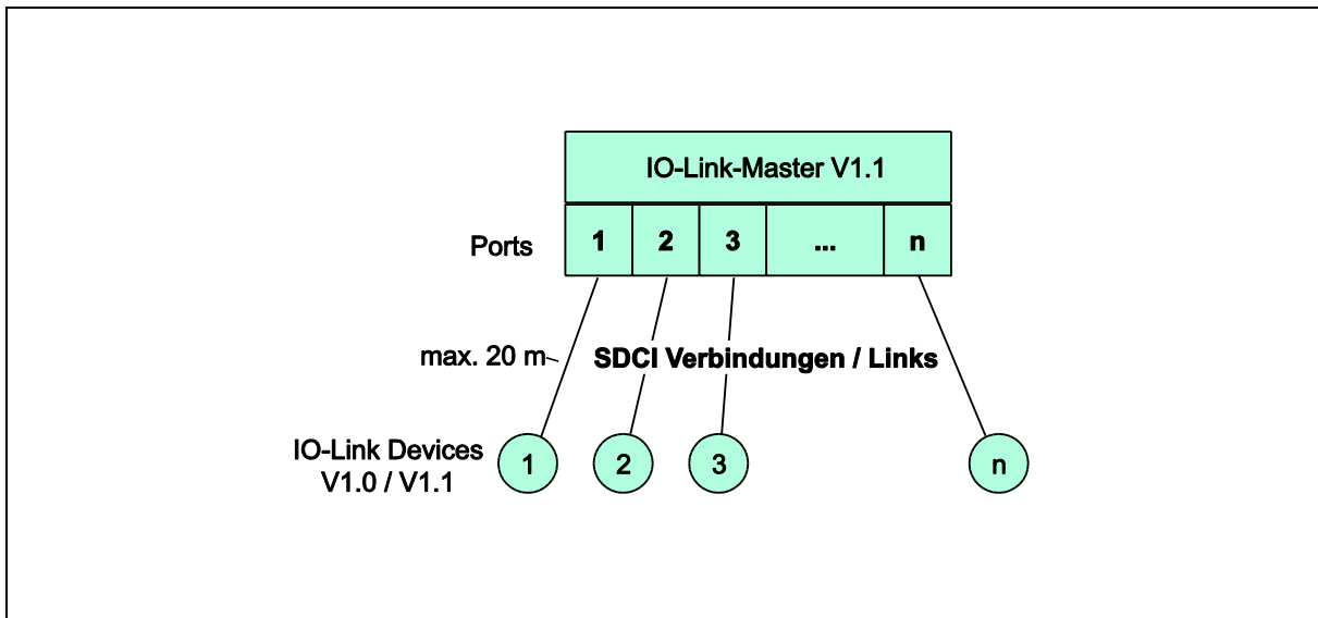
Abbildung 2: SDCI Topologie
