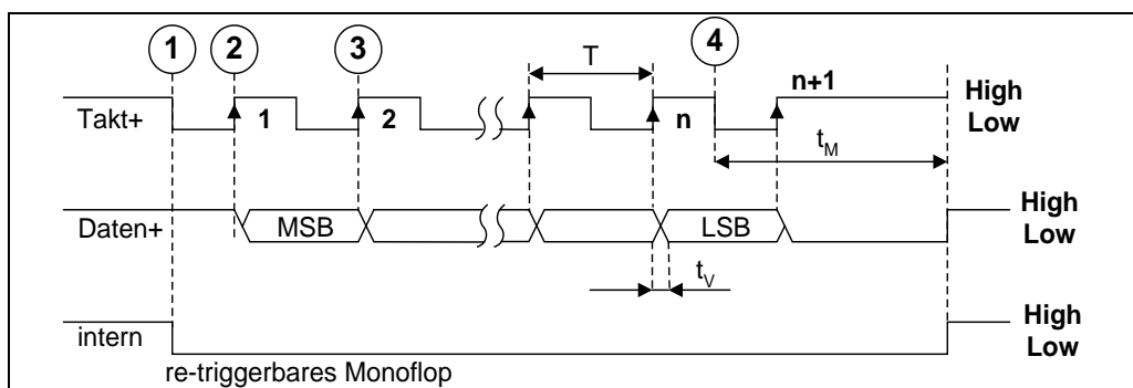
Abbildung 4: SSI-Übertragungsformat
