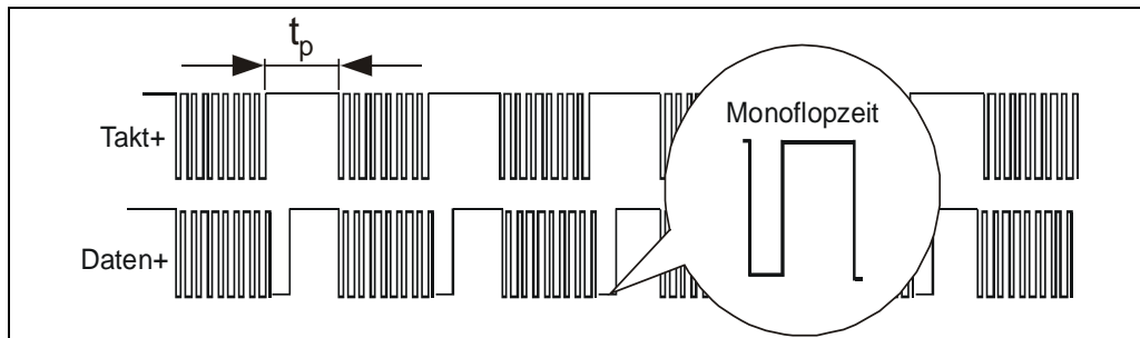
Abbildung 3: Typische SSI-Übertragungssequenzen
