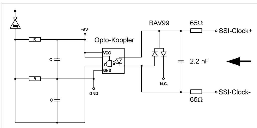
Abbildung 1: SSI Prinzip-Eingangsschaltung
