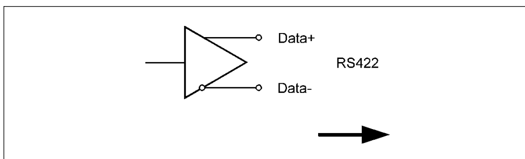
Abbildung 2: SSI-Ausgangsschaltung
