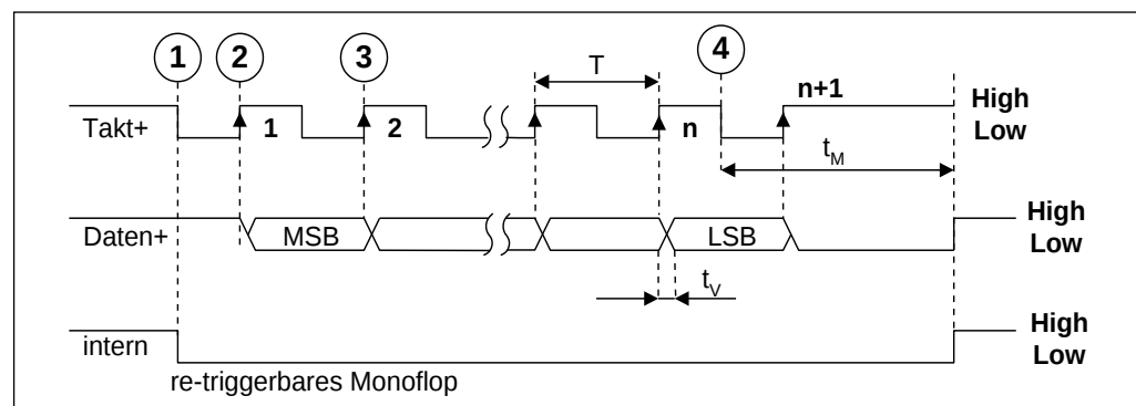
Abbildung 4: SSI-Übertragungsformat
