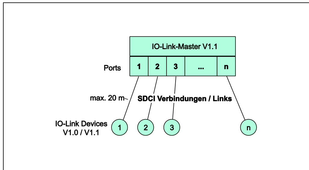
Abbildung 2: SDCI Topologie
