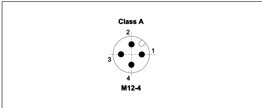
Abbildung 3: M12-Stecker, A-kodiert
