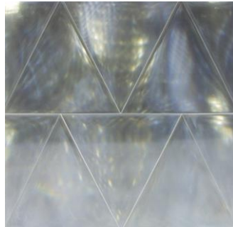
Fresnel
