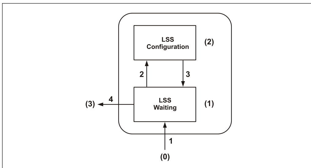
Abbildung 7: LSS FSA Zustandsmaschine
