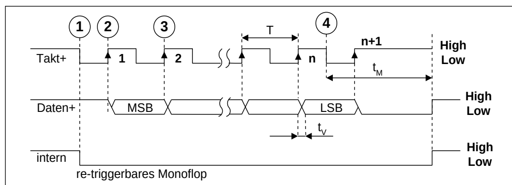
Abbildung 5: SSI-Übertragungsformat
