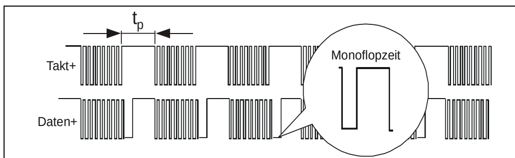
Abbildung 4: Typische SSI-Übertragungssequenzen
