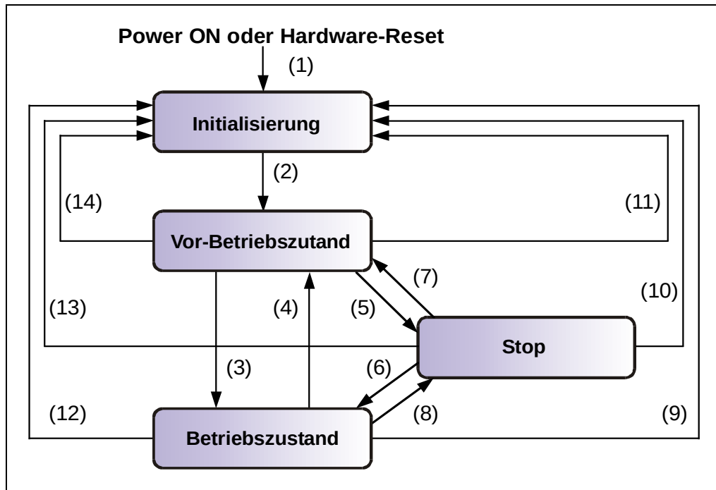
Abbildung 6: Boot-Up-Mechanismus des Netzwerkmanagements
