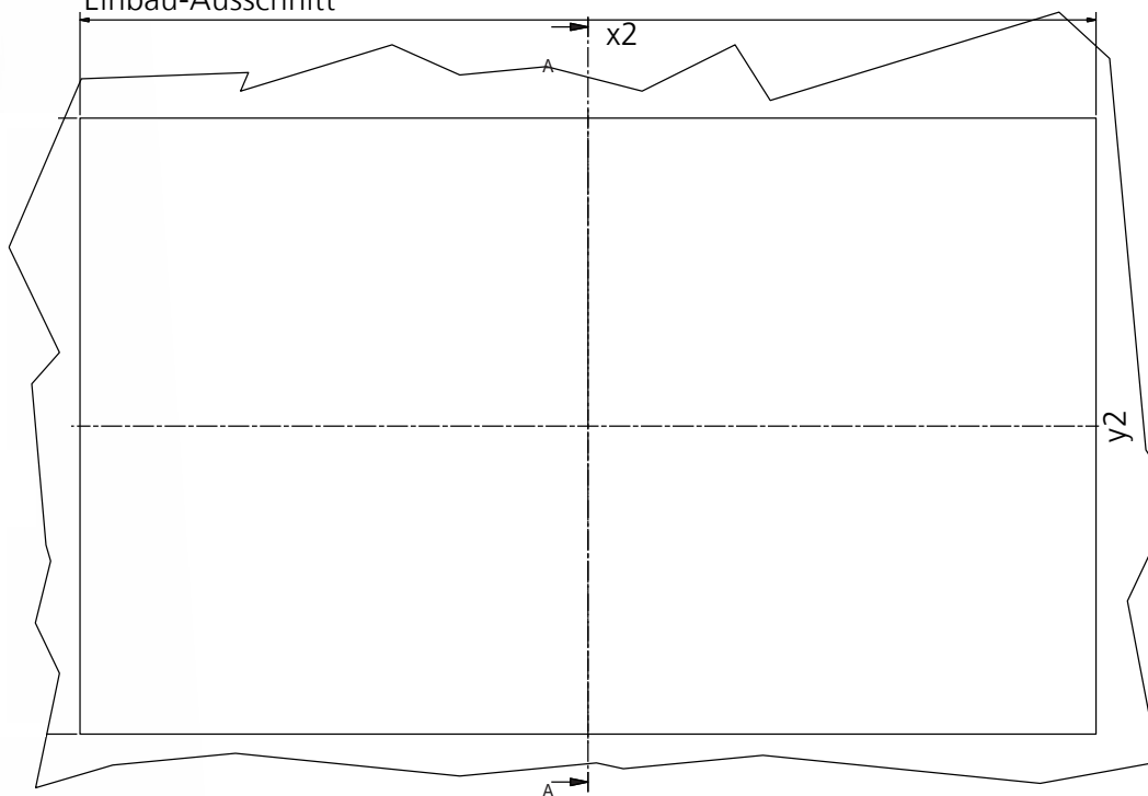
Einbau-Ausschnitt
